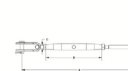
TURNBUCKLE,PIPE(SWIVEL TOGGLE+SWAGE TERMINAL),SS304 OR SS316. CSJX03
