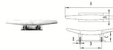
Cleat 底板式索栓
