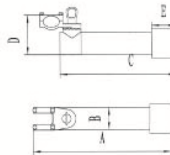
旋转鱼杆座
