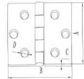
合页
