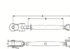
TURNBUCKLE,PIPE(SWIVEL TOGGLE+SWAGE TERMINAL),SS304 OR SS316. CSJX03
