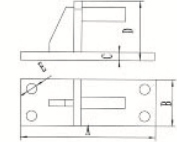
Hinge 铰链
