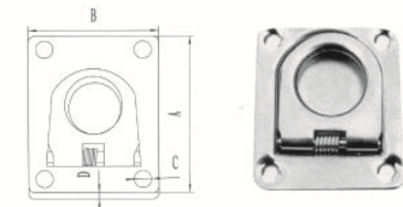
Lift Ring 地板扣
