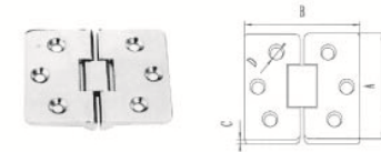
Hinge 合页
