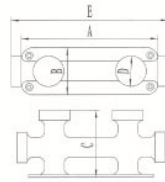
双十字缆桩
