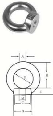
EYE NUT DIN582,CSLM02
