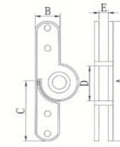
Padeyes
