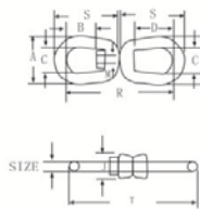
US TYPE SWIVEL G-402 美式旋转环G-402
