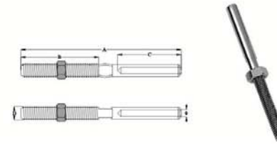
STUD TERMINAL, SS304 OR SS316. CSJX12
