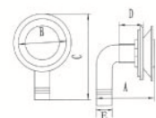
Air Vent 油箱透气口
