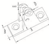
Deck Hinge 90° 栓式正山型座
