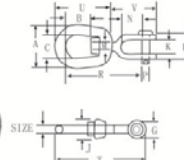
US TYPE SWIVEL G-403 美式旋转环G-403
