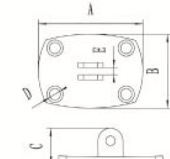
Deck Hinge 山型座
