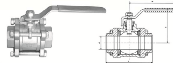
三片式球阀 3-PC BALL VALVE
