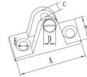
Heavy Duty Dety Hinge 90° 重山型座
