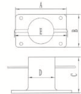
单十字缆桩
