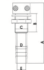
Air Vent 油箱透气口
