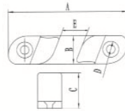
Bow Chocks 斜平导缆器
