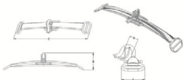
弧形座
