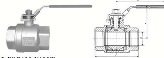
二片式球阀 2-PC BALL VALVE
