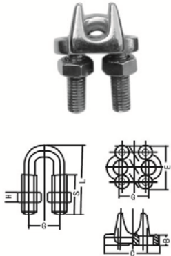
JIS TYPE WIRE ROPE CLIPS(日式卡头) CSKT02
