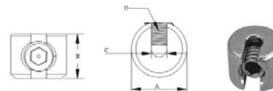
CABLE PIVOT,SS304 OR SS316.
