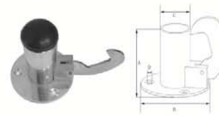
ROD TERMINAL(DOME),SS304 OR SS316.
